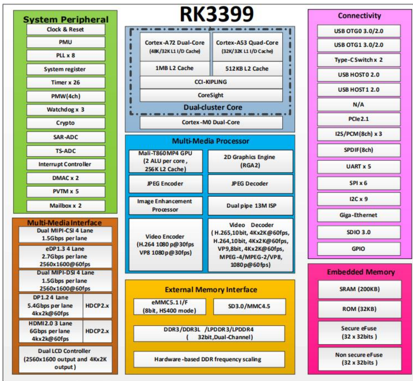
图 1 - 1 RK3399 框图
